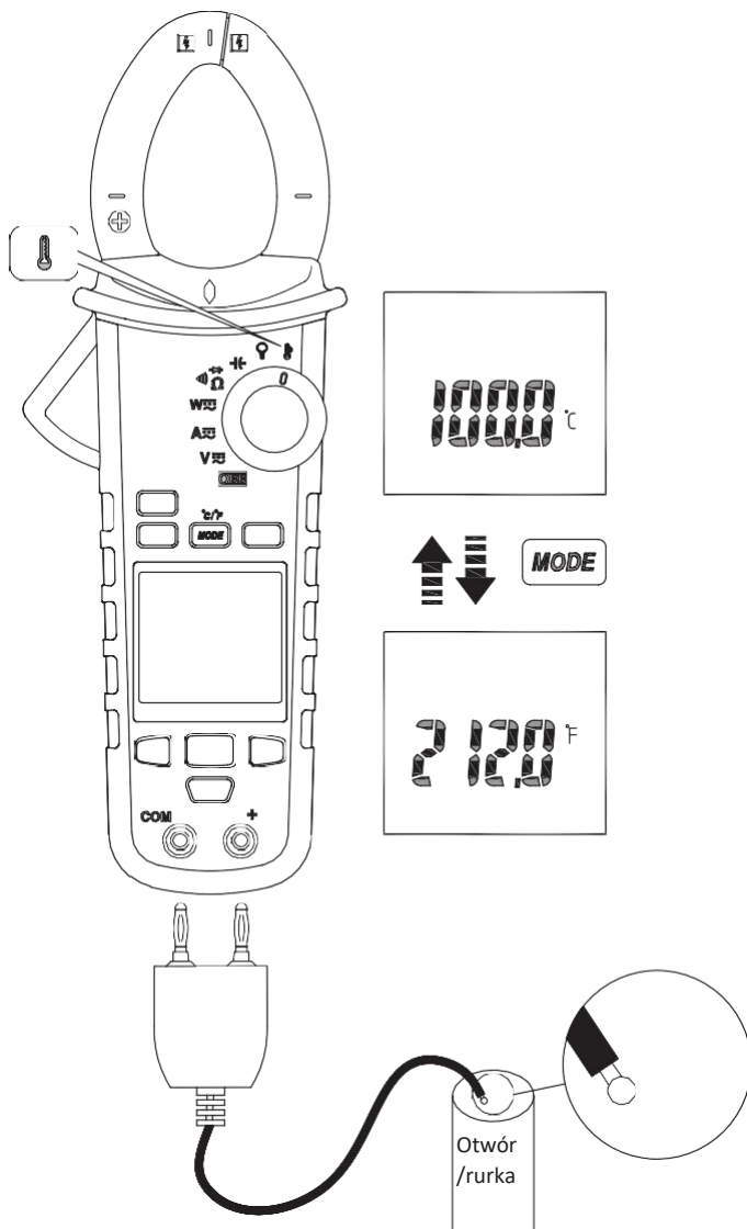
Termopara typu K
