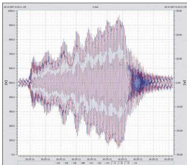
Obraz oscylograficzny
