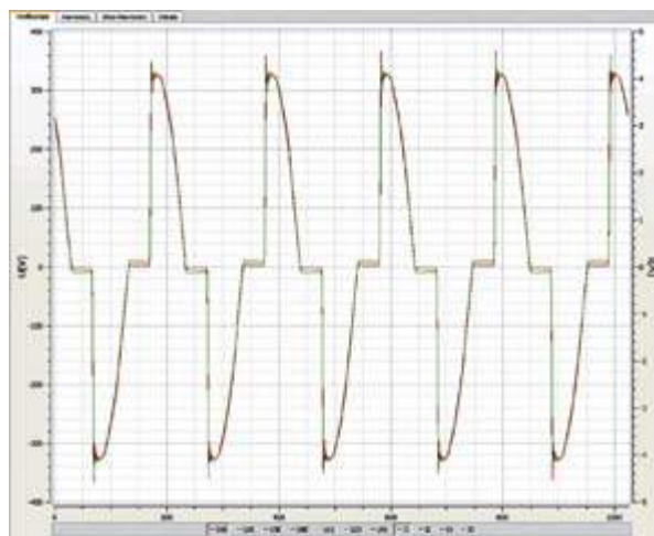
Oscyloskop online próbkowanie 41kHz
