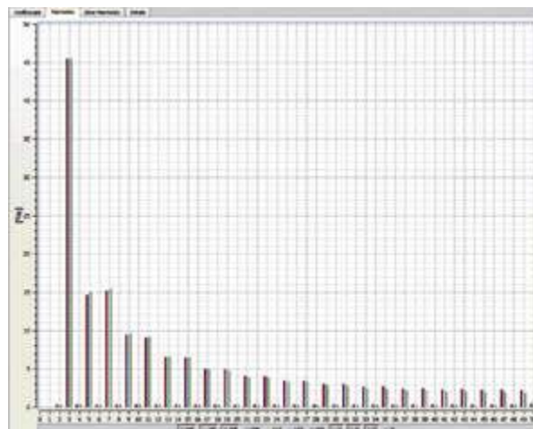
Harmoniczne online (napięcie i prąd do 9kHz).
